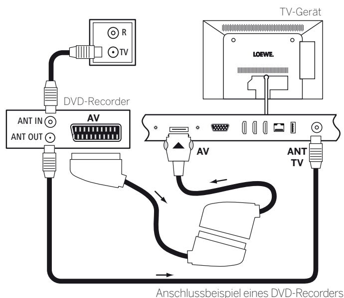
Anschlussbeispiel eines DVD-Recorders
