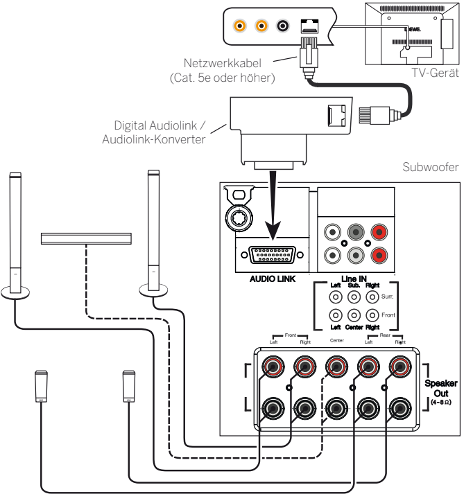
Anschluss des Loewe Lautsprechersystems an das TV-Gerät
