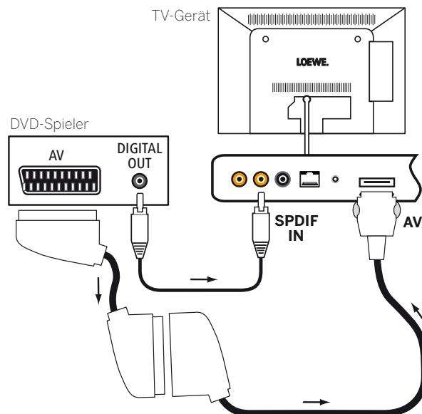
Anschlussbeispiel für einen DVD-Spieler
