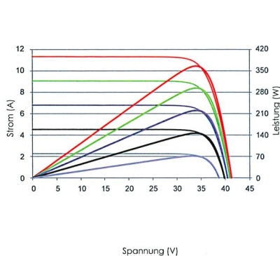
Strom-Spannungs- und Leistungs-Spannungskennlinien (365W)
